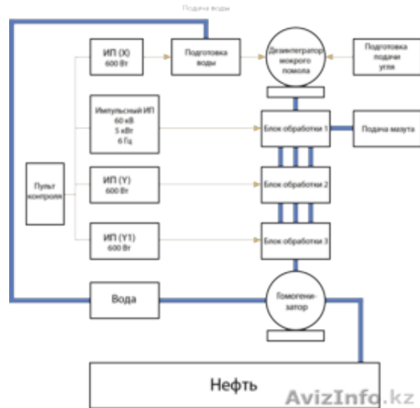
Установка по производству нефти из угля
